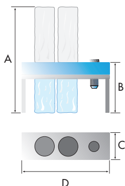
GRUPPO MONTATO - GROUPE MONTÉ ASSEMBLED UNIT - GERÄT MONTIERT - GRUPO MONTADO mm - inch
